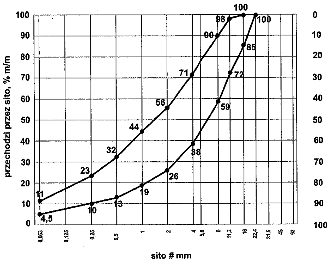
Rys. 1 Uziarnienie mieszanki CBGM 0/16
