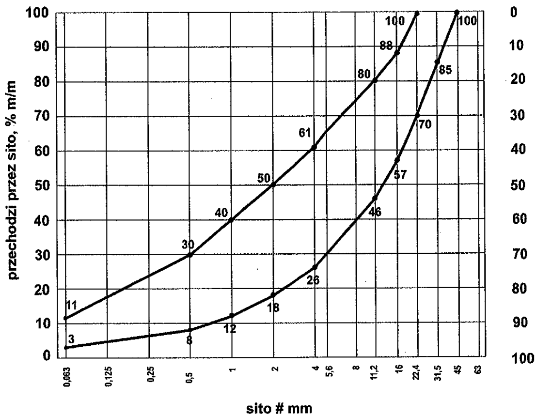
Rys. 2 Uziarnienie mieszanki CBGM 0/31.5
